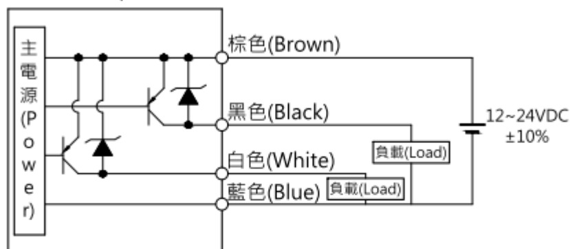
輸出模式 (Output) : PNP
