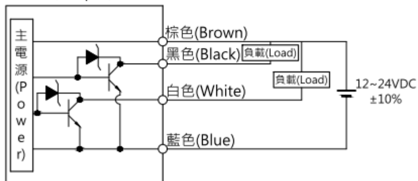
輸出模式 (Output) : NPN
